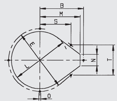
Ölbehälterdruchbruch
