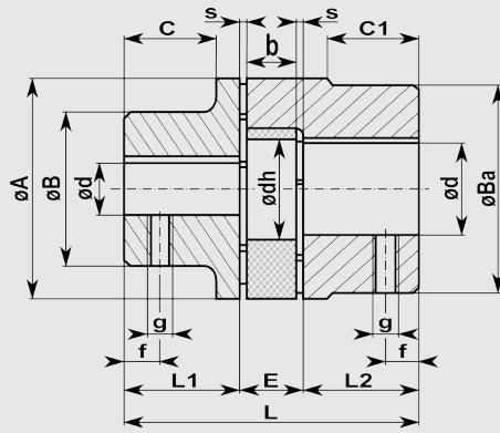
Nabenkombination A/B z.B. Kupplung 28/38 – 28/35
